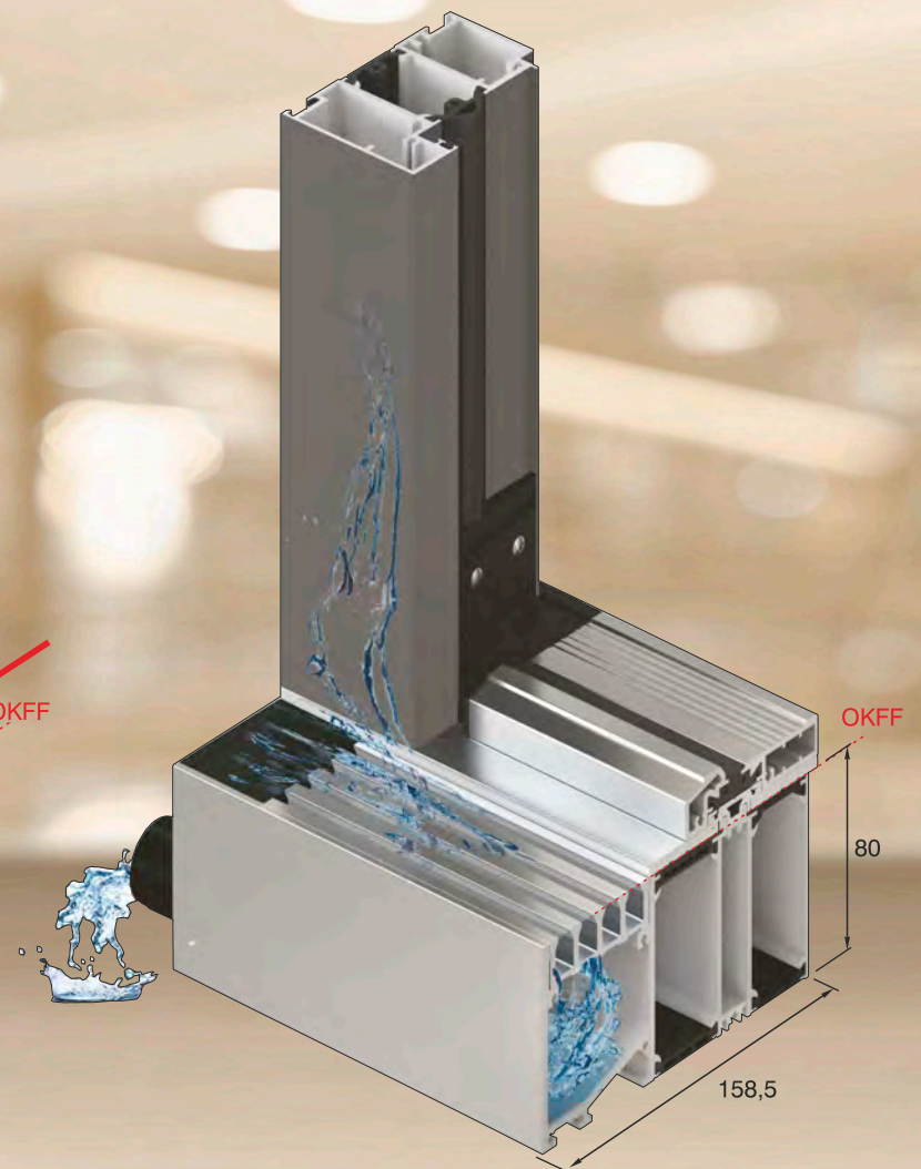
Entwässerungsrinne 80 mm
