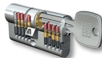
cylindrická vložka X-pert (standard)
